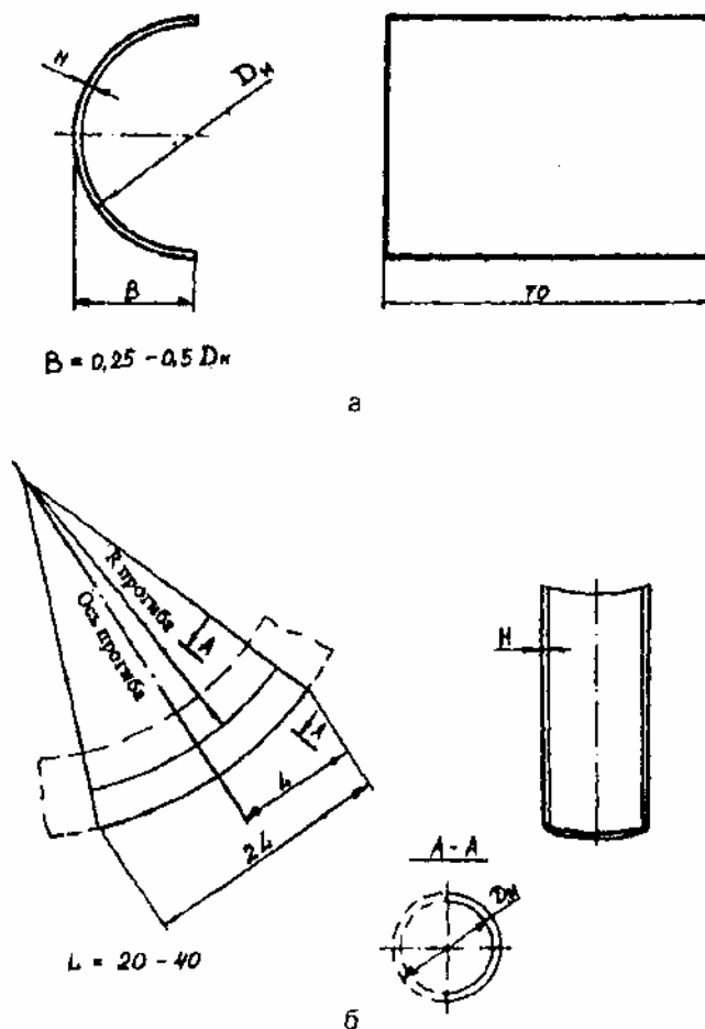
Рис. ПА.2- СОП в виде фрагментов изделий. а - отрезок трубы; б - участкагиба трубы; D_n - номинальный диаметр; Н - толщина стенки
